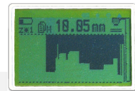
Barrido de piezas con representación grafica tipo B-Scan en tiempo real.
