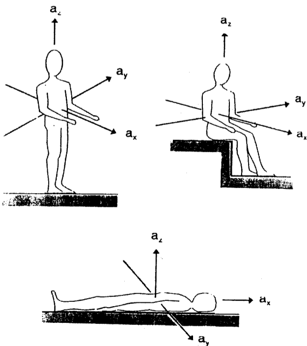
Figura 3: Sistema de coordenadas biodinámicas para medir las aceleraciones (adapado según ISO 2631). ax, ay, az = aceleración en la dirección de los ejes, x, y, z; eje x dirección espalda-pecho; eje y dirección derecha-izquierda; eje z dirección pies-cabeza.
